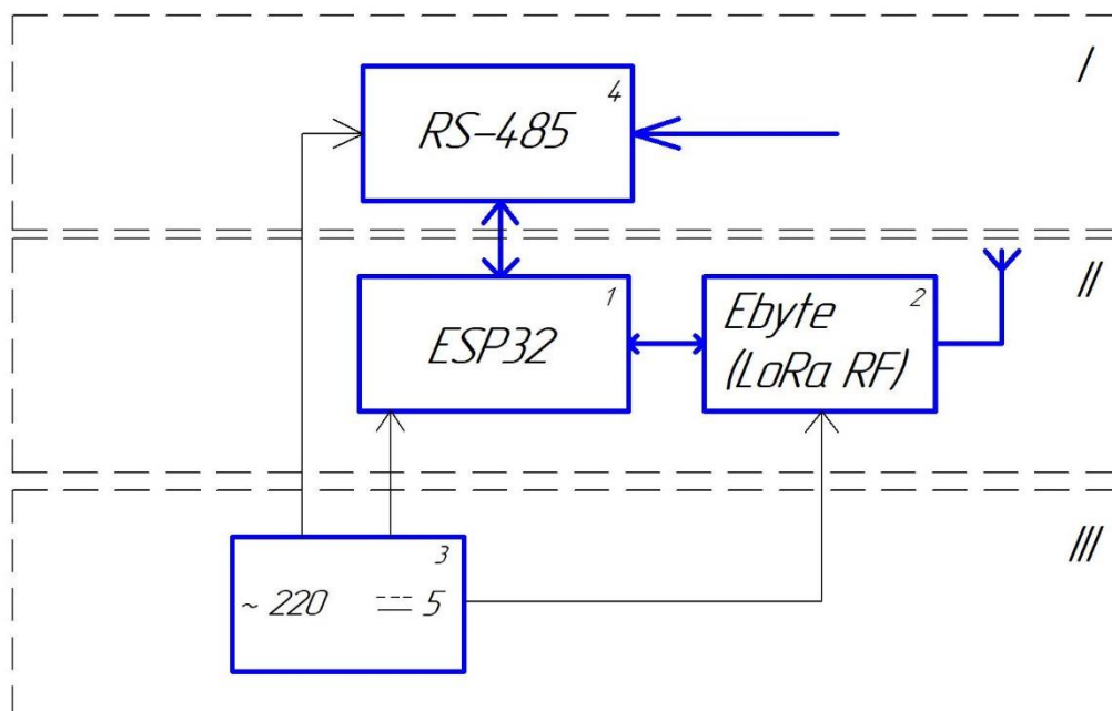
Рис. 1.1. Структурно-функціональна схема пристрою
