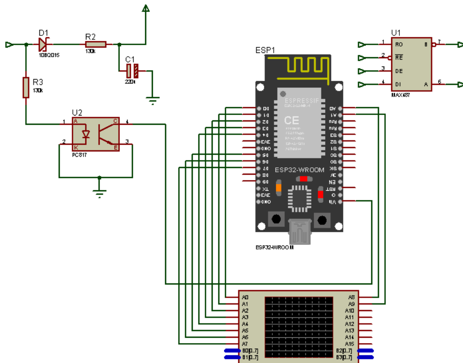
Рис. 3.1. Схемотехнічна модель пристрою
